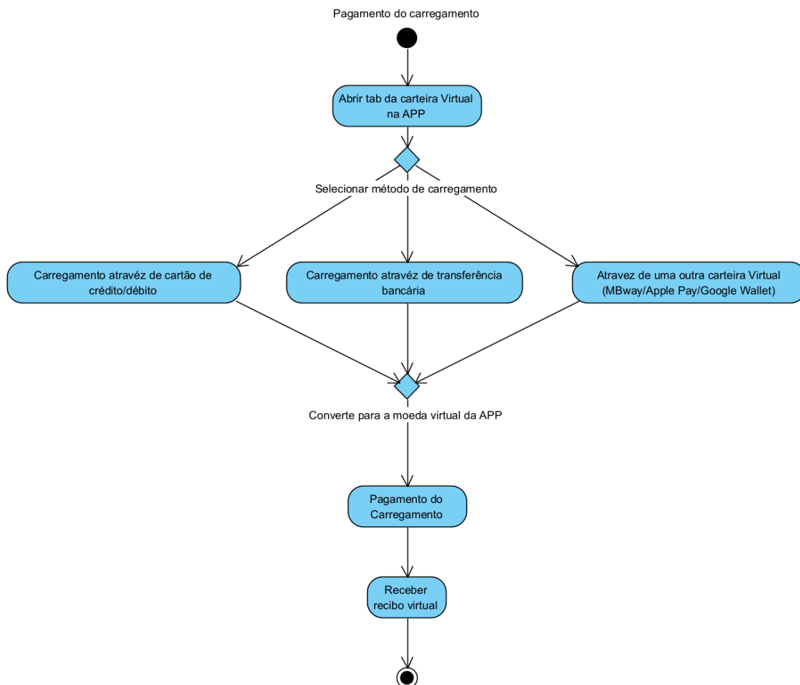
Fig.3: Diagrama de atividade do processo de unificação de métodos de pagamento
