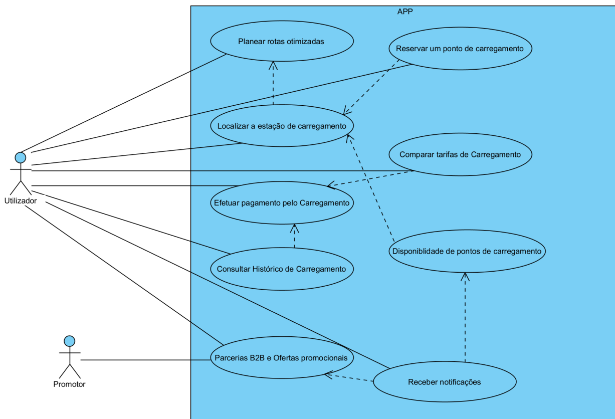
Fig.5: Diagrama de Casos de Utilização
